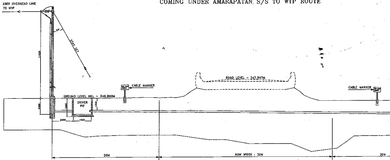
LONGITUDINAL SECTION
